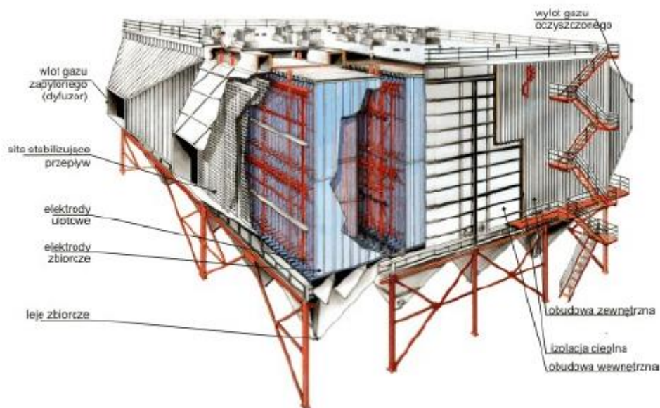
Rys. 5.5. Elektrofiltr przemysłowy – rysunek zaczerpnięty z pracy [13]
