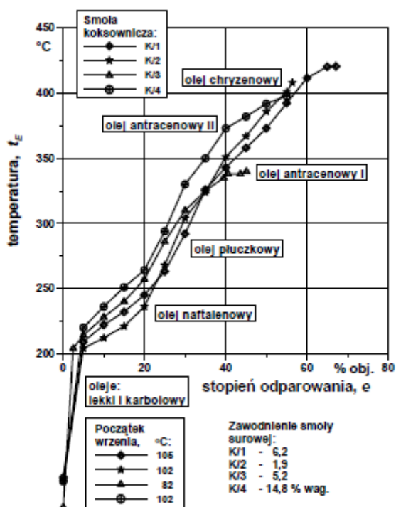
Rys. 5.3. Krzywe wrzenia smoly koksowniczej, wg [18, 19]
