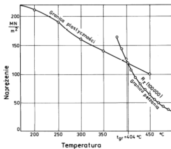
Rys. 5.4. Wytrzymałość stali St41K w podwyższonej temperaturze, wg [21]
