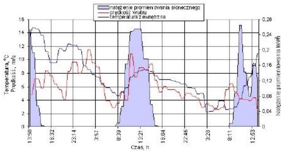
Rys. 5.2. Charakterystyka czasowa parametrów środowiska
