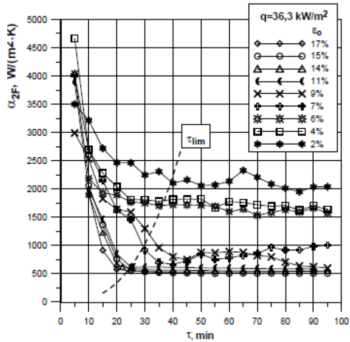
Rys. 5.1. Wpływ czasu na wartość współczynnika wnikania ciepła
